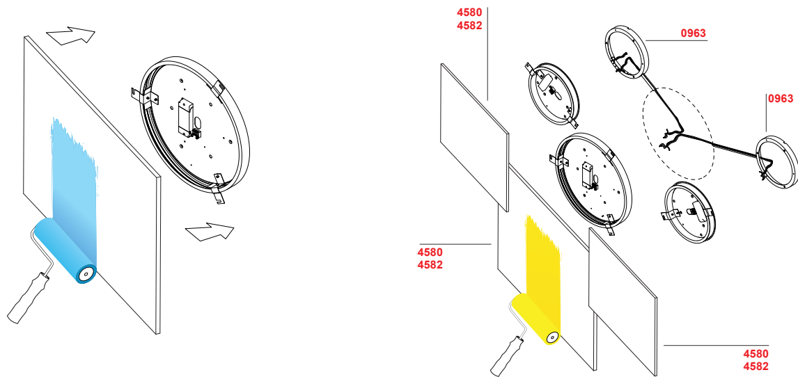
Esempio di installazione singola Example of single installation
