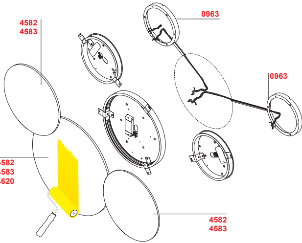
Esempio di installazione multipla con distanziali Example of multiple installation with spacers Art.4620 può essere utilizzato in installazioni multiple purché sia posizionato come lampada sulla parete. Art.4620 can be used in multiple installations as long as it is positioned as a lamp on the wall.
