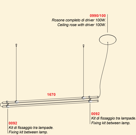
Kit di fissaggio a sospensione fornito con la lampada. - Suspension fixing kit supplied with the lamp.
