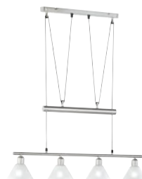
Pendelleuchte · Pendant ↔ 80 x 14 cm, ↑ 80 - 180 cm excl. 4 x E14, max. 40 W
