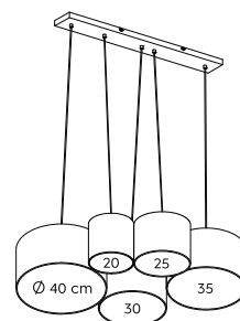
Pendelleuchte · Pendant ↔ 96,5 x 68,5 cm, ↓ 150 cm excl. 5 x E27, max. 42 W
