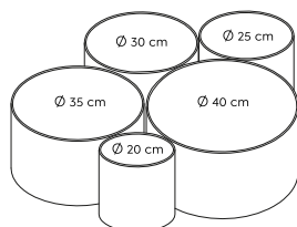
Deckenleuchte · Ceiling lamp ↔ 90 x 70 cm, ↑ 21,5 cm excl. 5 x E27, max. 42 W
